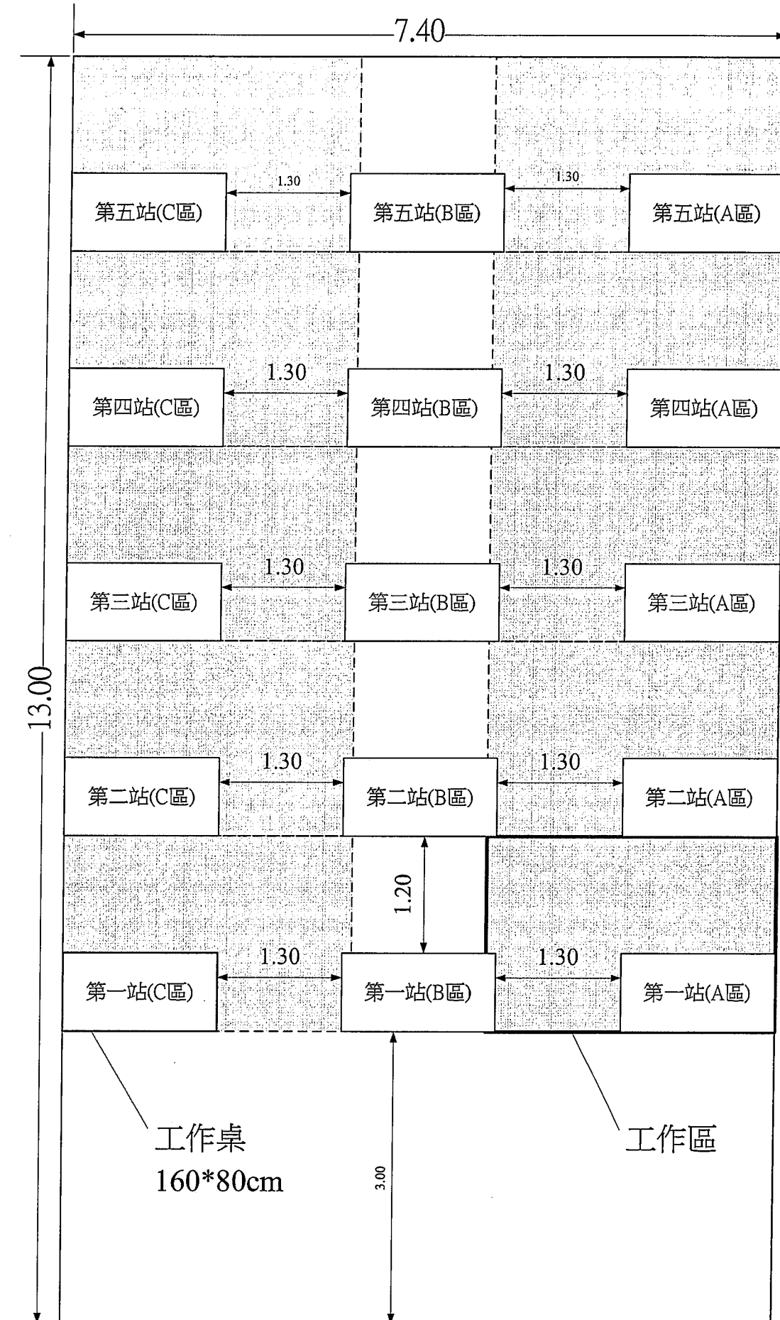
健行科技大學 電機工程系 機電整合工廠配置圖
