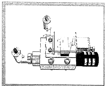
(11)真空產生器含壓力開關
