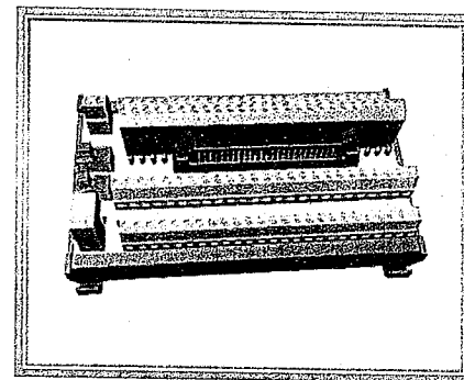
(11)端子台附排線座
