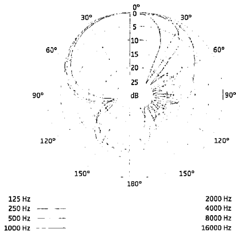
▲指向圖
